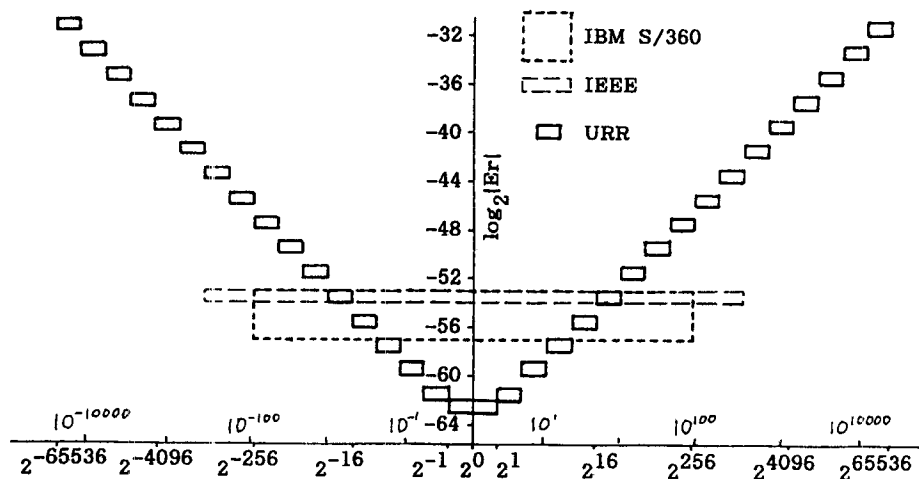
Fig.2 Er over wide range.
